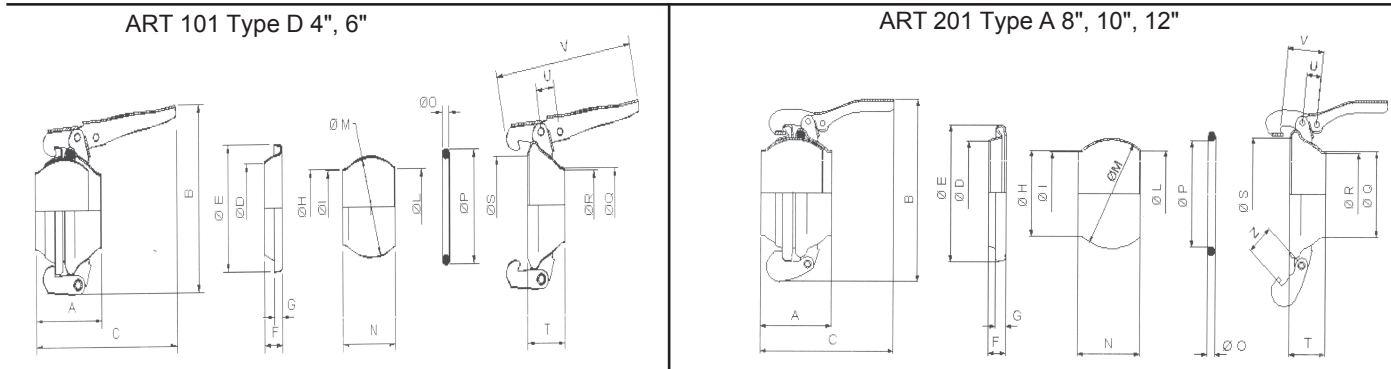
ART 101 Type D 4", 6" ART 201 Type A 8", 10", 12"
