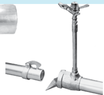
Sprinkler
